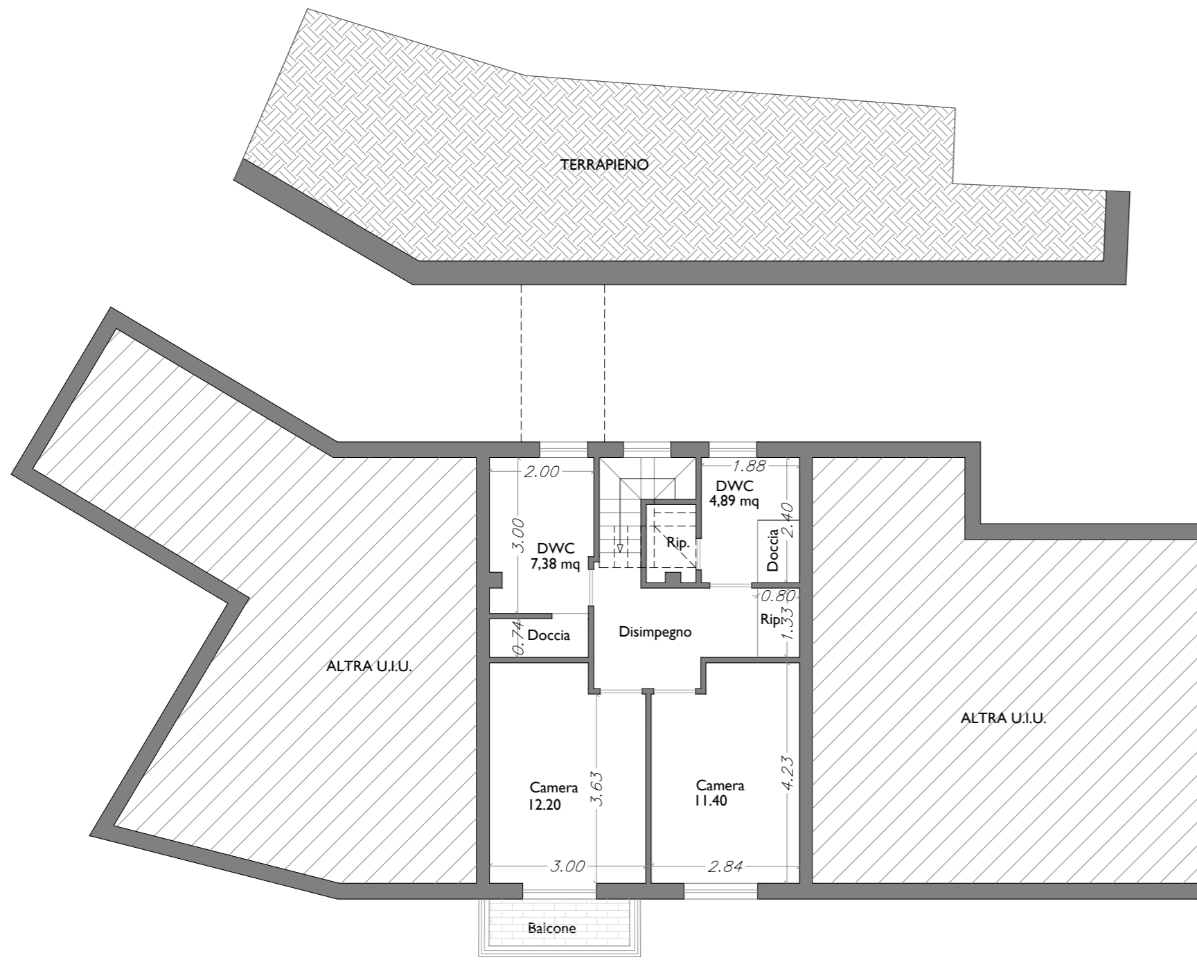
PLANIMETRIA PIANO TERRENO
