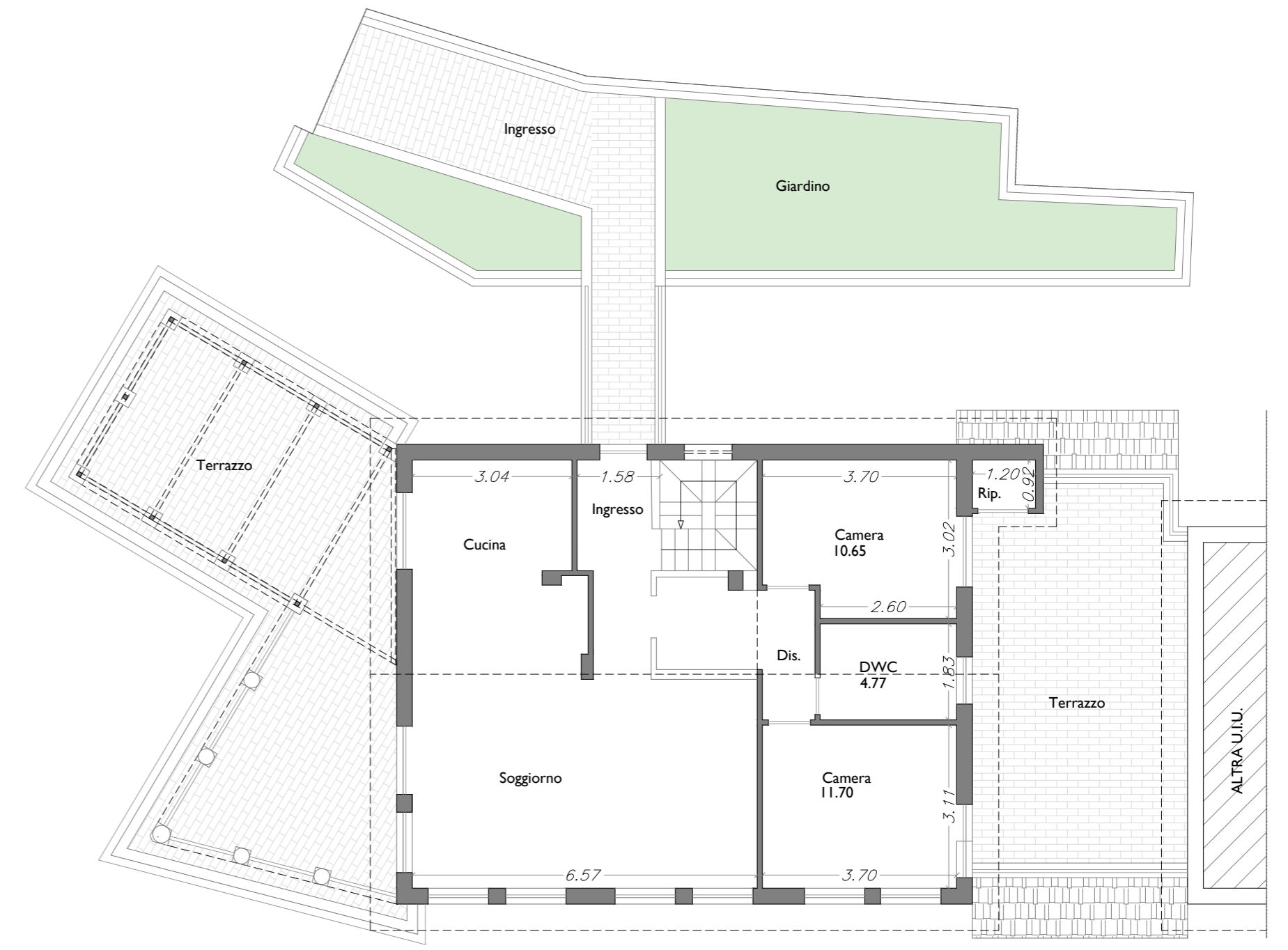
PLANIMETRIA PIANO PRIMO
